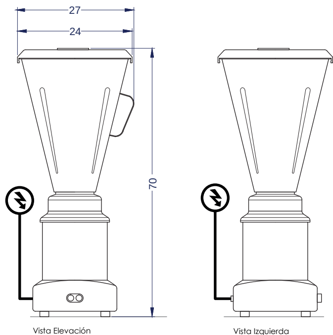
Vista Elevación
